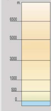
Capas Hipso Batimétricas
