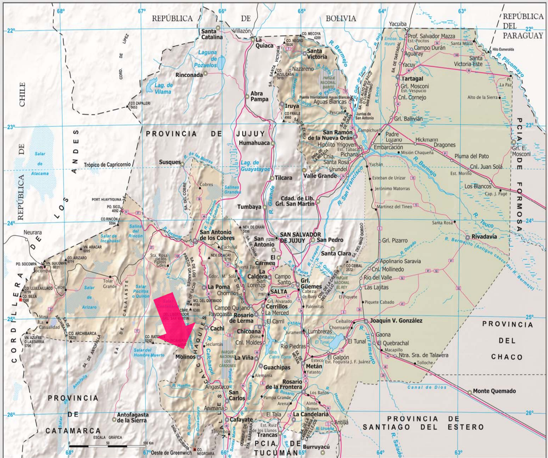
Capas Hipso Batimétricas
